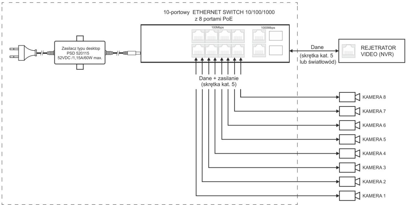
Rys. 1. Schemat blokowy.
