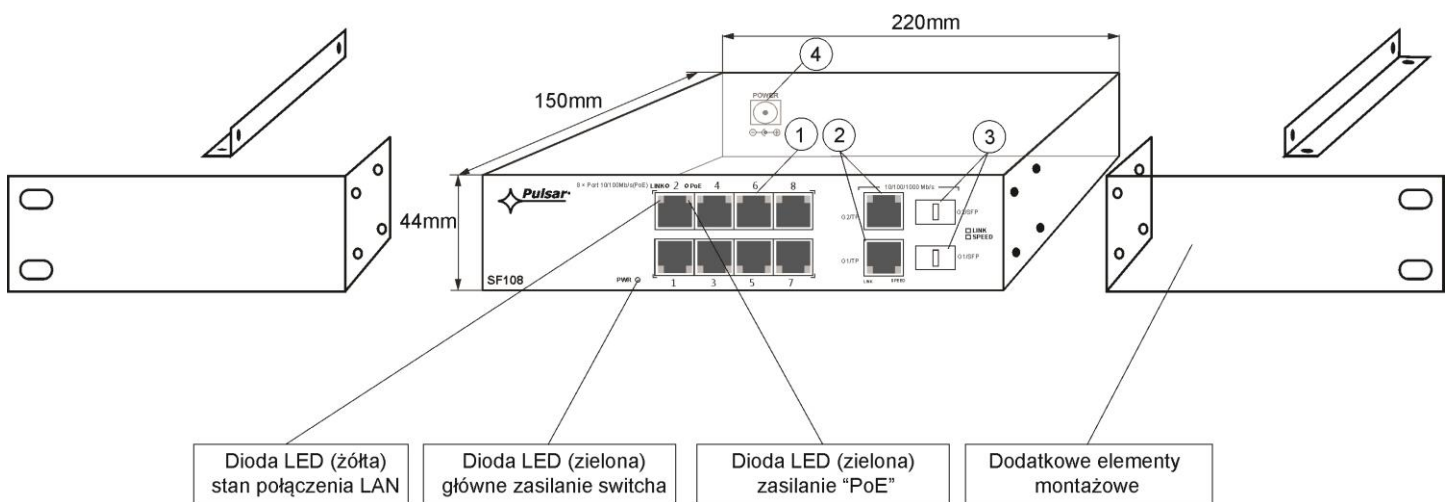
Rys. 2. Widok switch'a.
