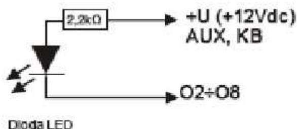
Wyjście O2-O4 : podłączenie diody LED, zasilanie +12V= AUX.
