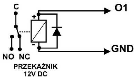
Wyjście O1: podłączenie przekaźnika 12V DC.
