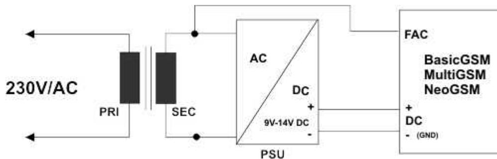
Wejście FAC podłączenie kontroli napięcia AC (po transformatorzez separacyjnym).
