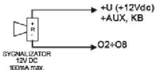
Wyjście O2-O4: podłączenie sygnalizatora 12VDC/100mA max. (akustycznego i/lub optycznego).
