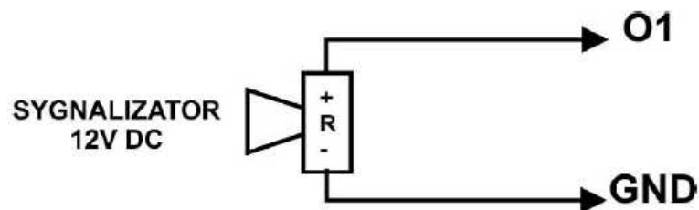
Wyjście O1: podłączenie sygnalizatora 12V DC (akustycznego i/lub optycznego).
