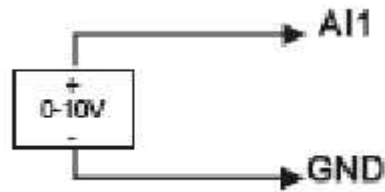
Wejście AI podłączenie źródła napięciowego.
