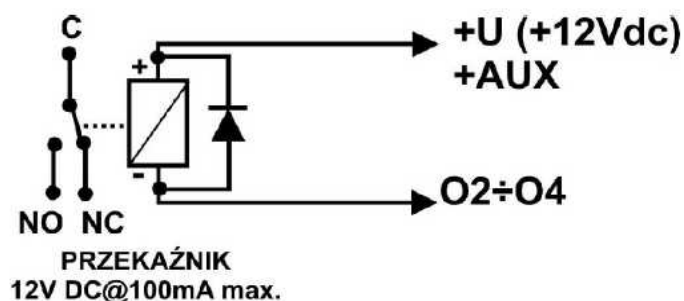
Wyjście O3-O8: podłączenie przekaźnika 12V DC, zasilanie +12V= AUX.
