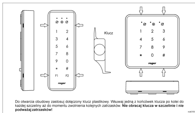
Rys. 3 Sposób otwarcia obudowy czytników PRT82MF i PRT84MF
