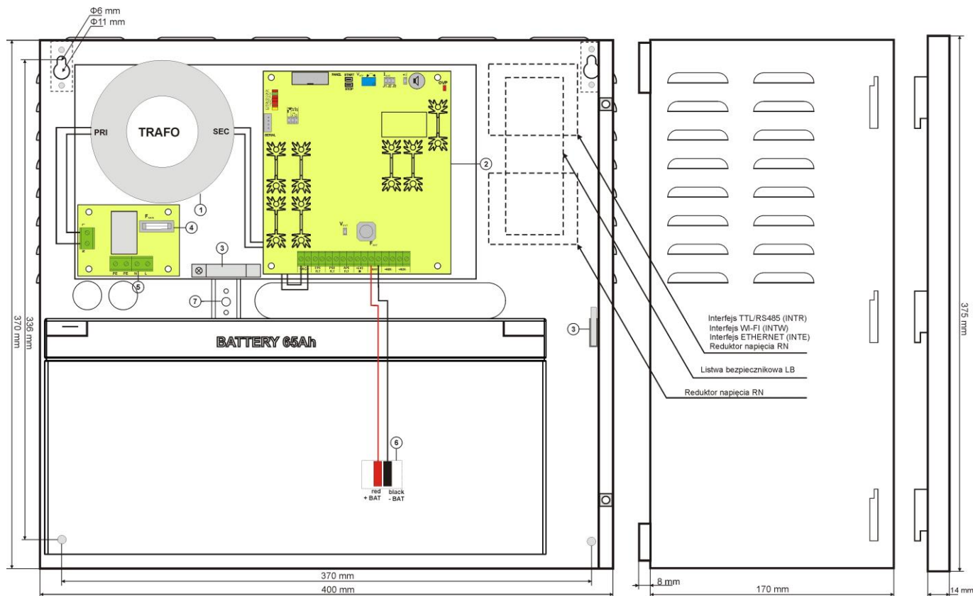
Rys.3. Widok zasilacza.
