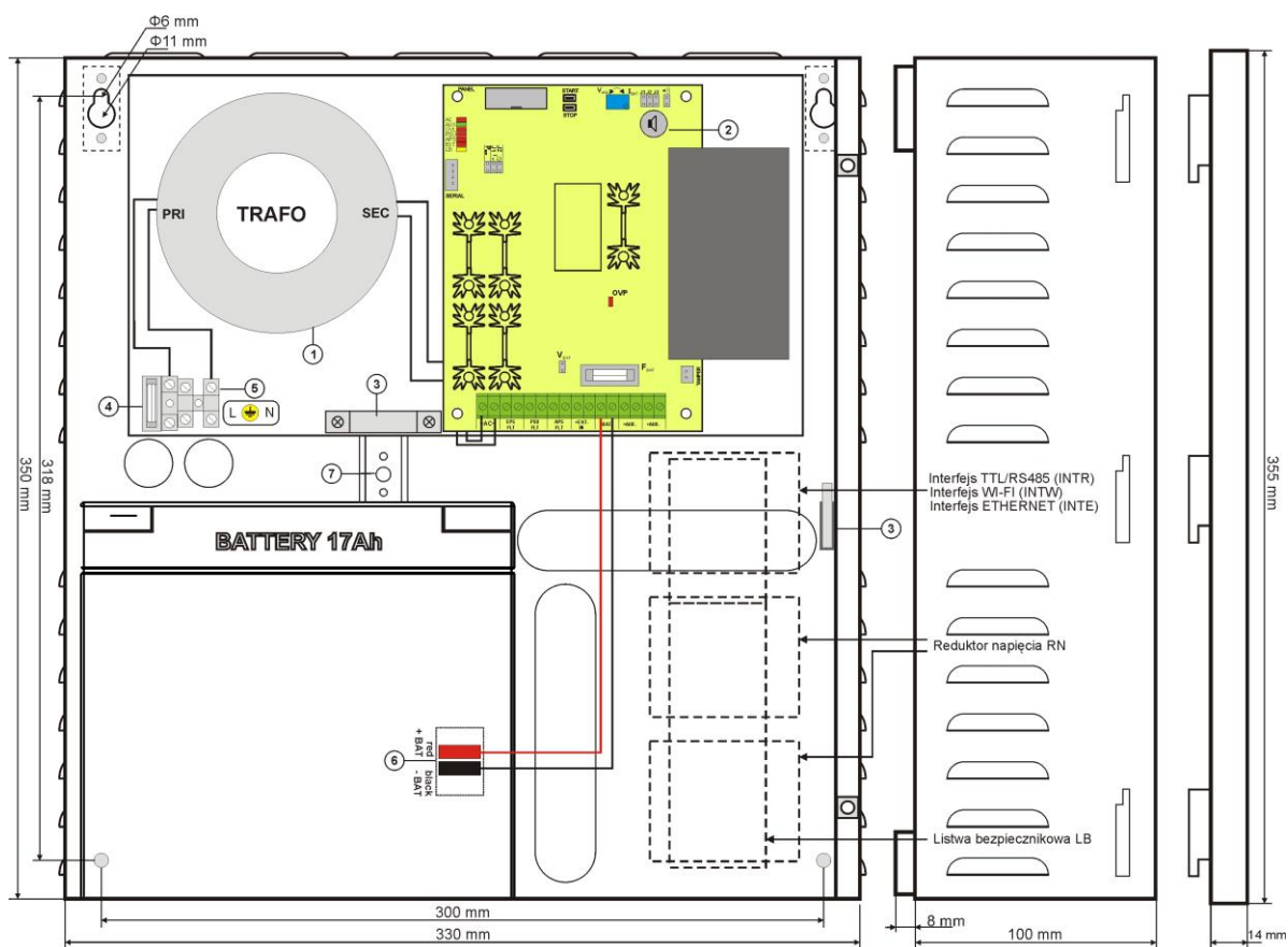
Rys.3. Widok zasilacza.
