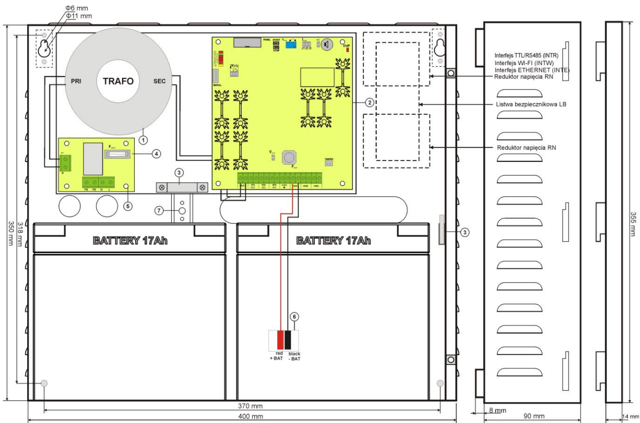
Rys.3. Widok zasilacza.
