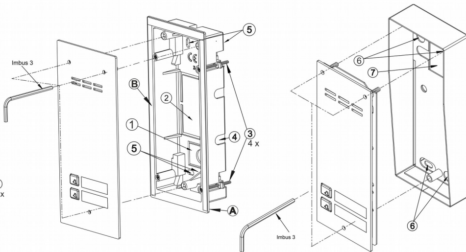
Rys. 5 Montaż paneli podtynkowych
