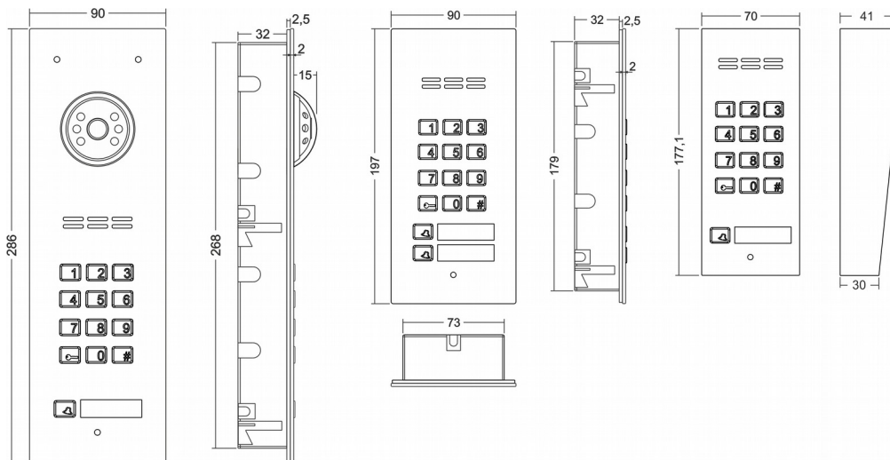
Rys. 7 Wymiary paneli
