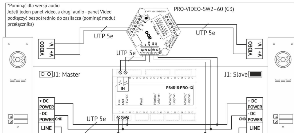
Rys. 2 Przykładowy schemat podłączenia panelu w systemie wideo.
