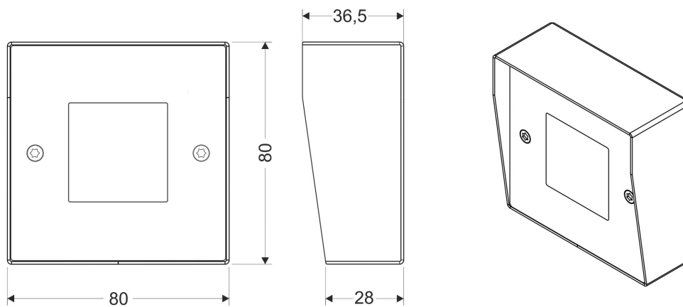
Wersja natynkowa / Surface-mounted version
