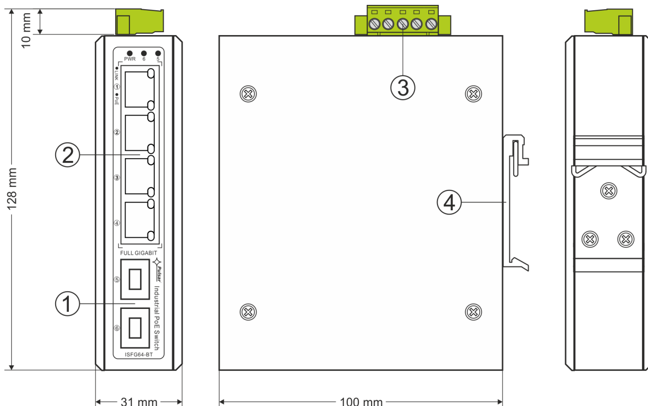
Rys. 2. Widok switch'a.
