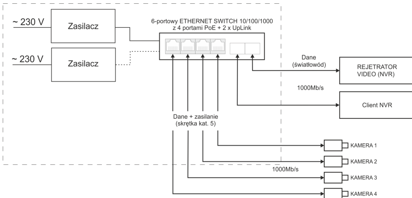
Rys. 1. Schemat blokowy.
