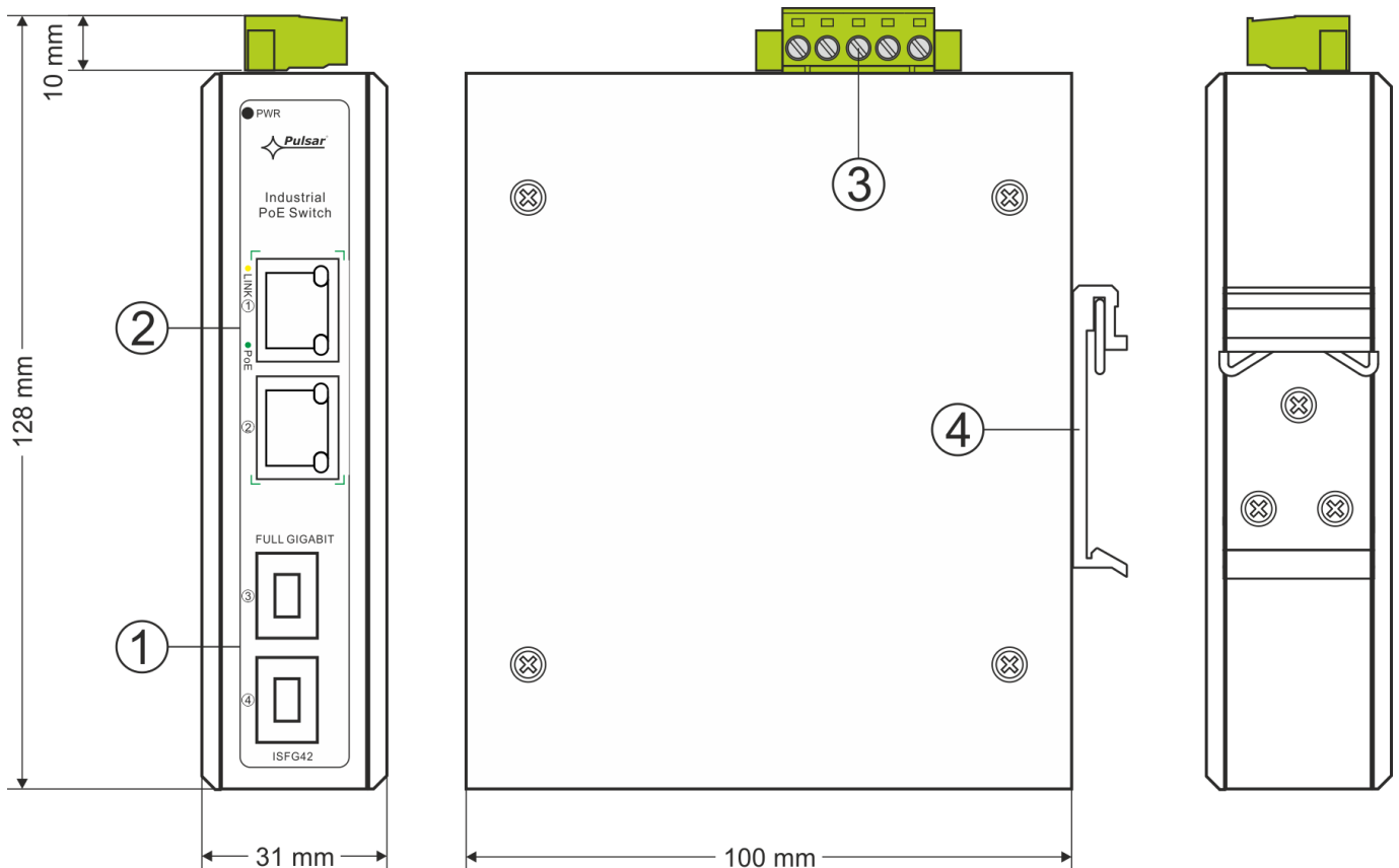
Rys. 2. Widok switch'a.
