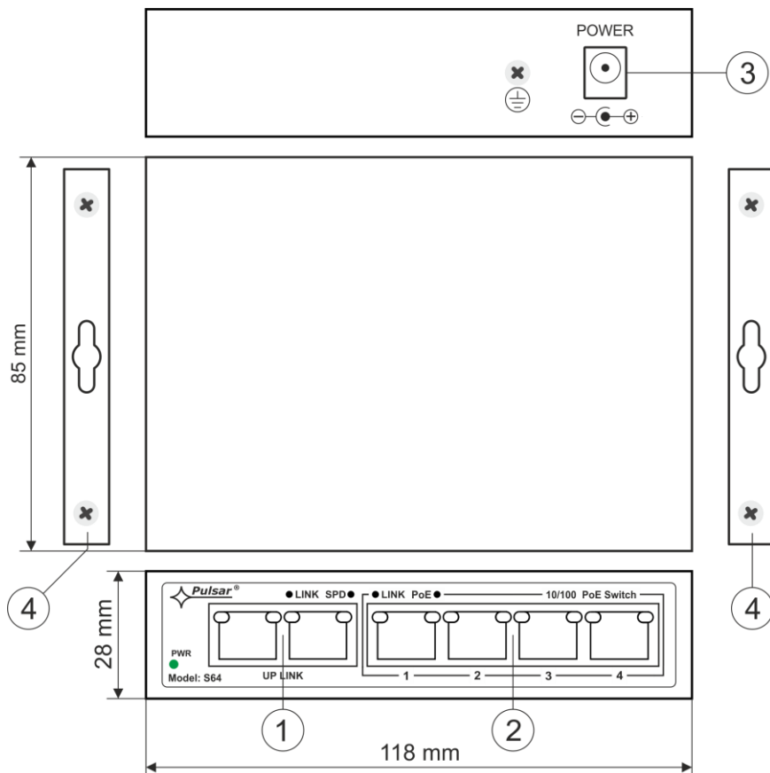
Rys. 2. Widok switch'a.
