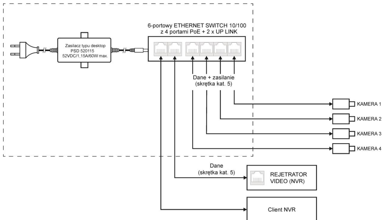
Rys. 1. Schemat blokowy.
