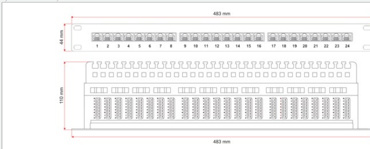
Rysunek techniczny
