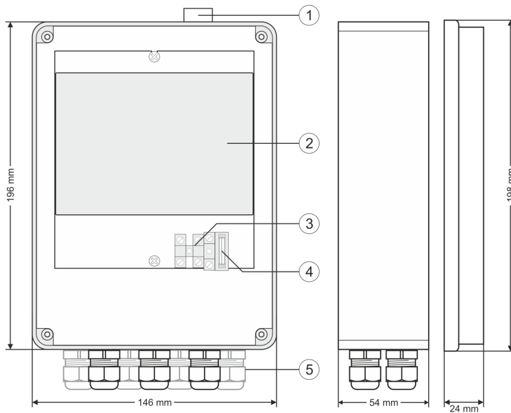
Rys. 2. Widok obudowy.
