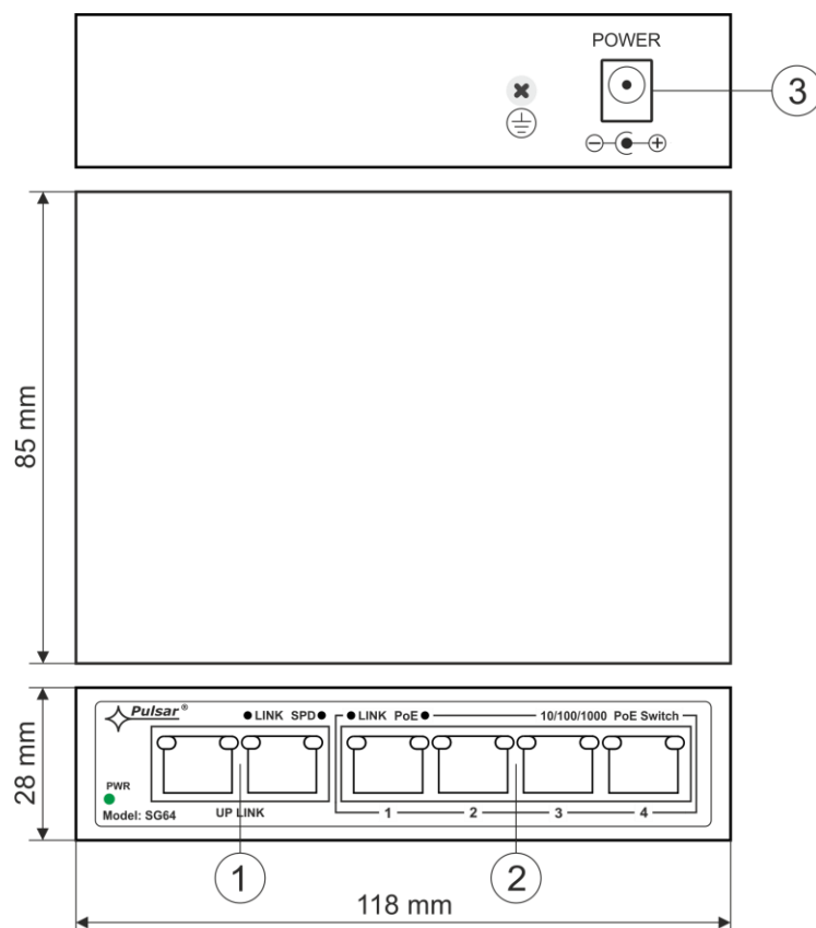
Rys. 3. Widok switch'a.
