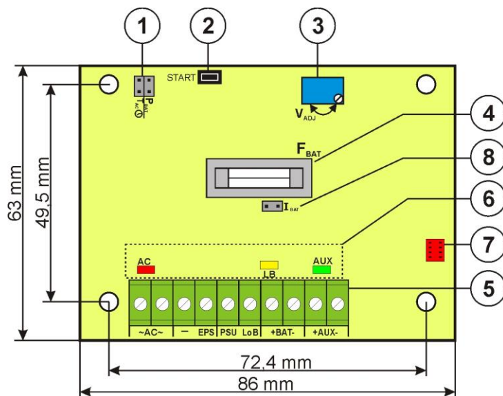
Rys. 2. Widok płyty pcb modułu zasilacza.
