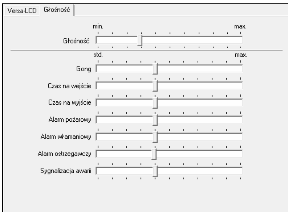
Rys. 16. Program DLOADX: konfigurowanie głośności manipulatora.
