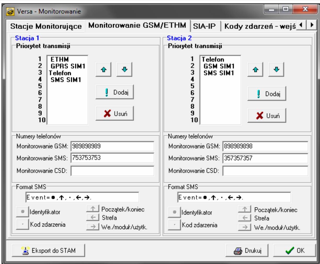
Rys. 23. Program DLOADX: zakładka „Monitorowanie GSM/ETHM” w oknie „Versa – Monitorowanie”.
