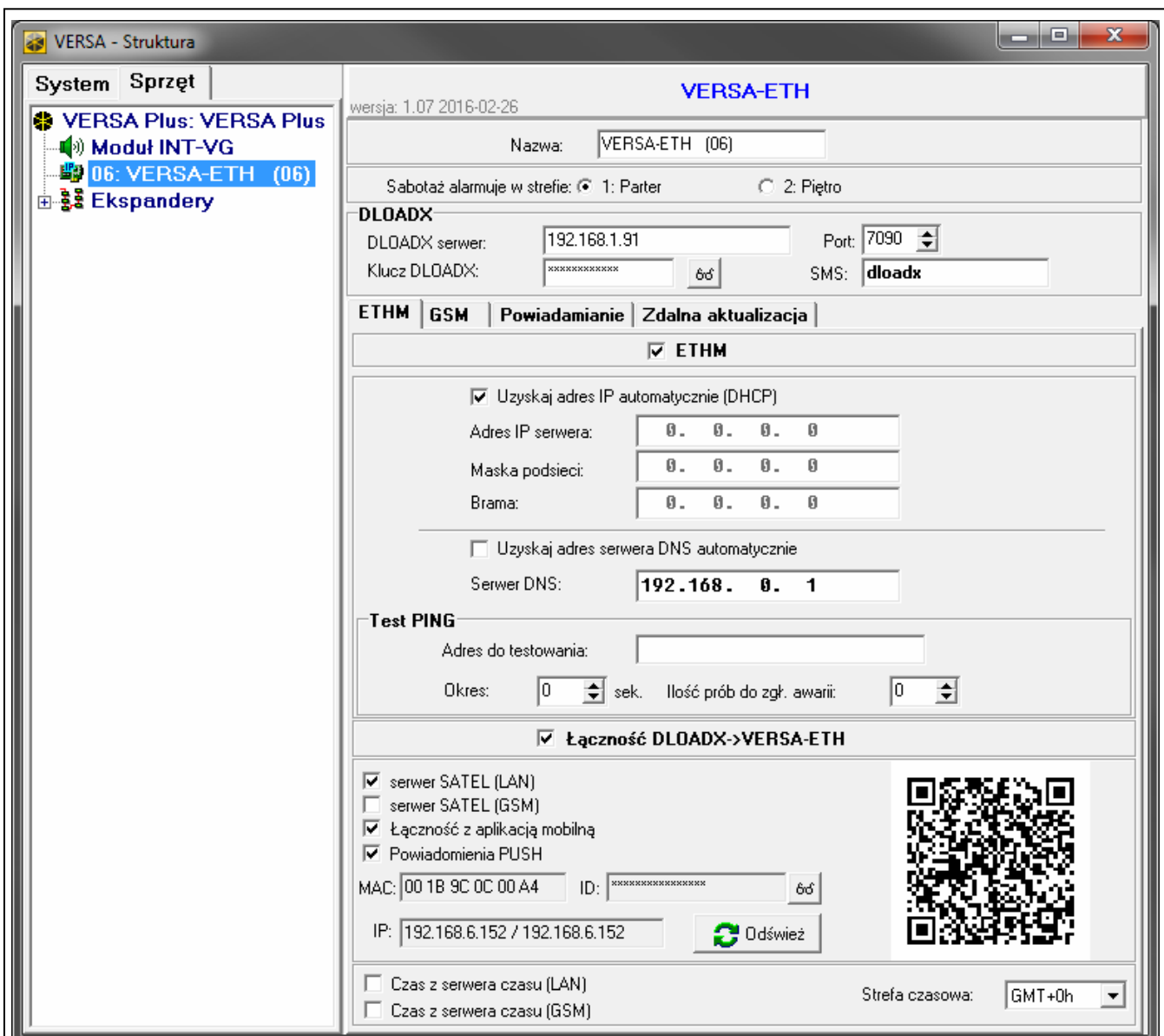
Rys. 13. Program DLOADX: konfigurowanie wbudowanych modułów komunikacyjnych.
