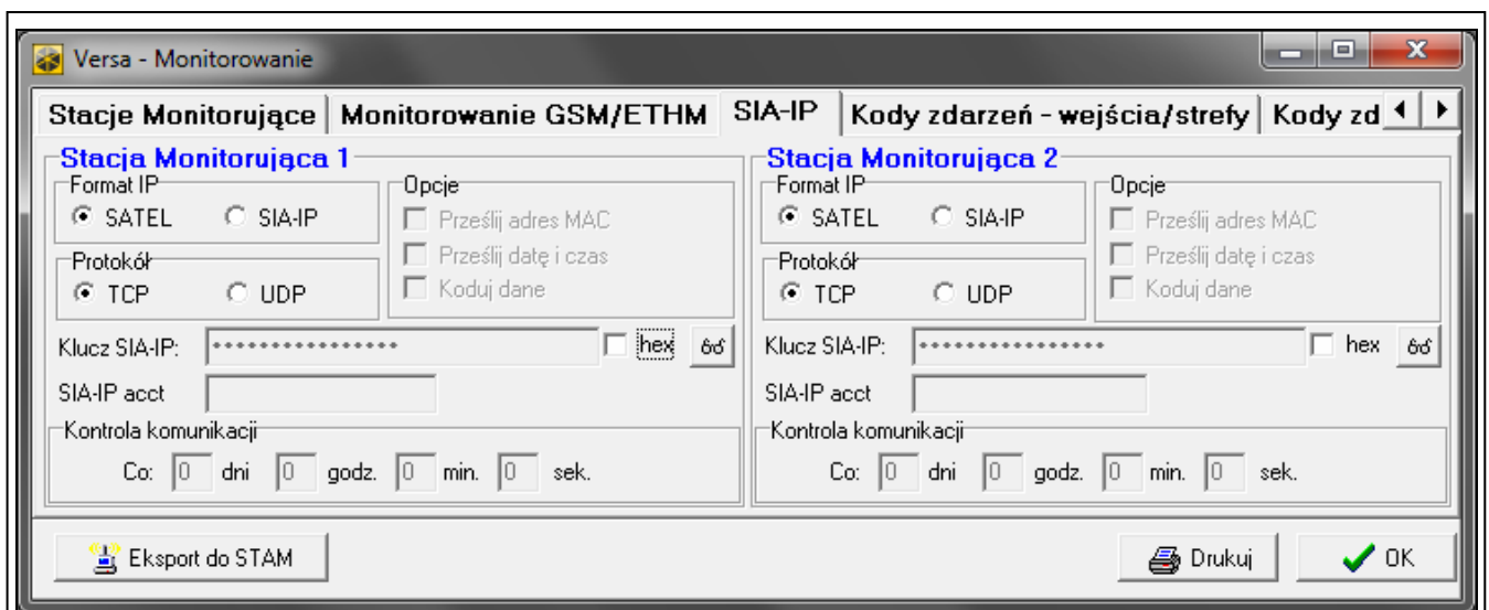
Rys. 24. Program DLOADX: zakładka „SIA-IP” w oknie „Versa – Monitorowanie”.
