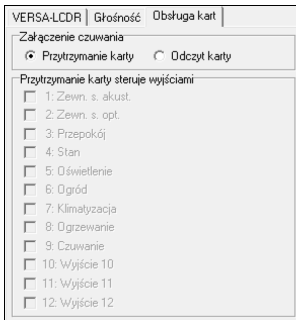
Rys. 17. Program DLOADX: konfigurowanie obsługi przy pomocy kart zbliżeniowych.
