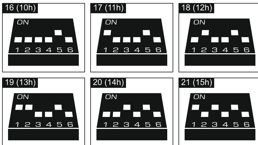
Rys. 16. Sposób ustawienia adresu na przykładzie modułu INT-IT / INT-IT-2.
